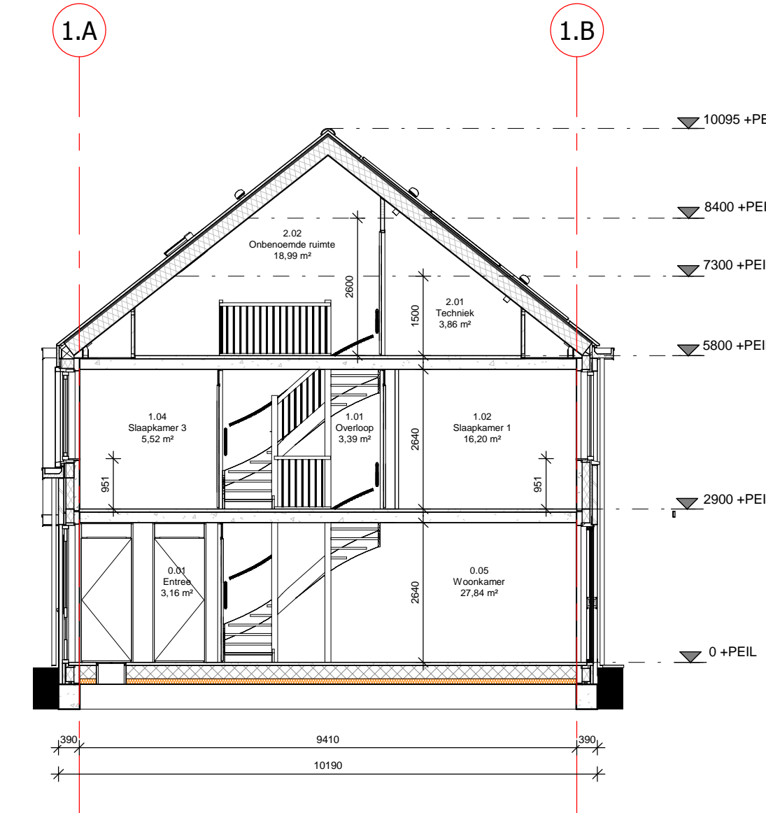
doorsnede 03_A
