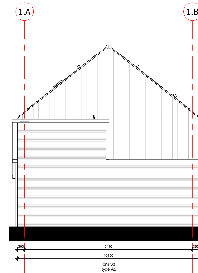
rechter zijgevel
