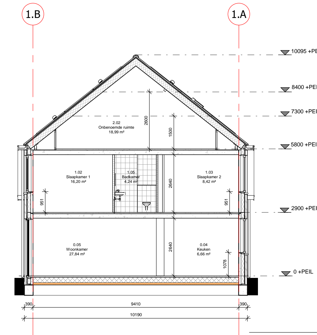
doorsnede 03_B
