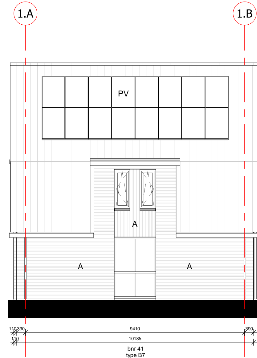
rechter zijgevel
