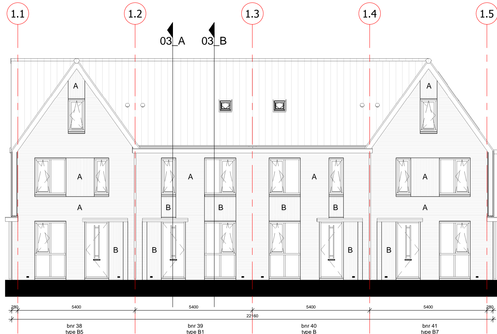
voorgevel
