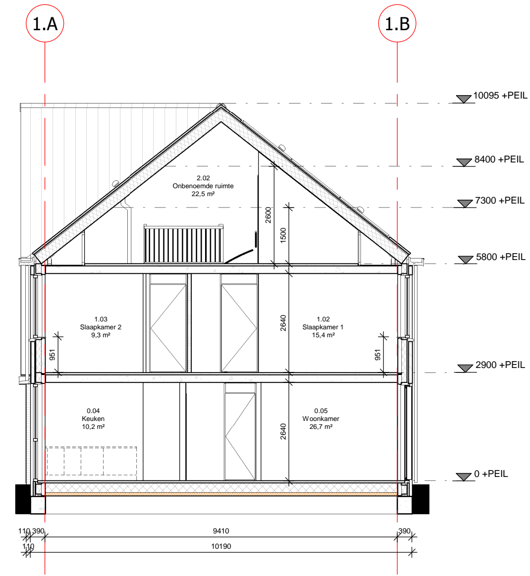
doorsnede 03_B
