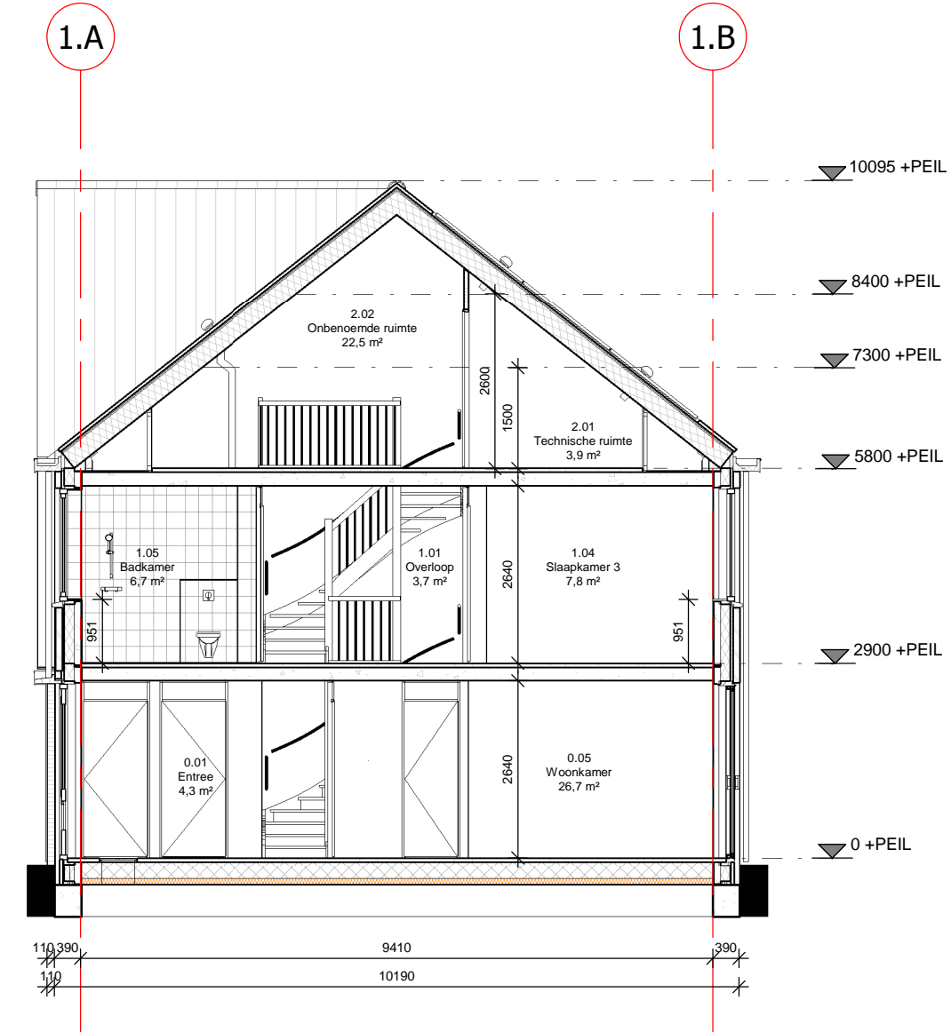
doorsnede 03_A
