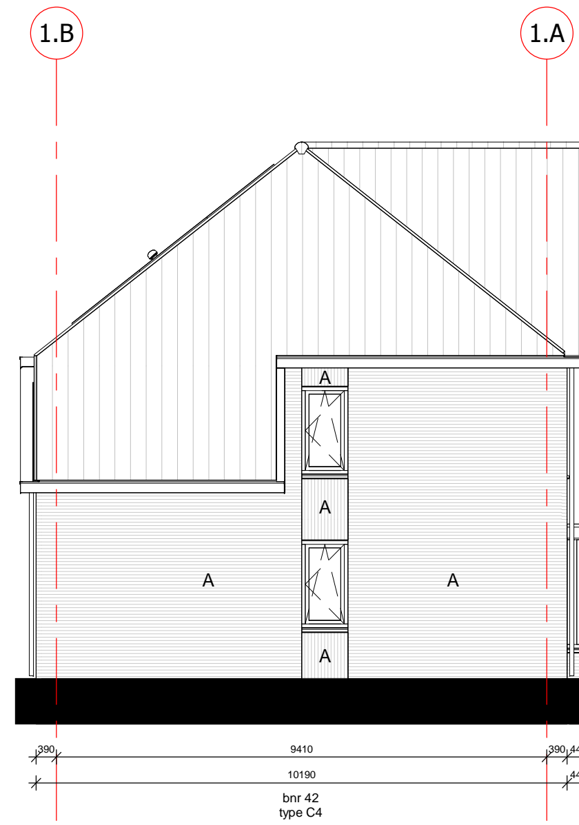
linker zijgevel
