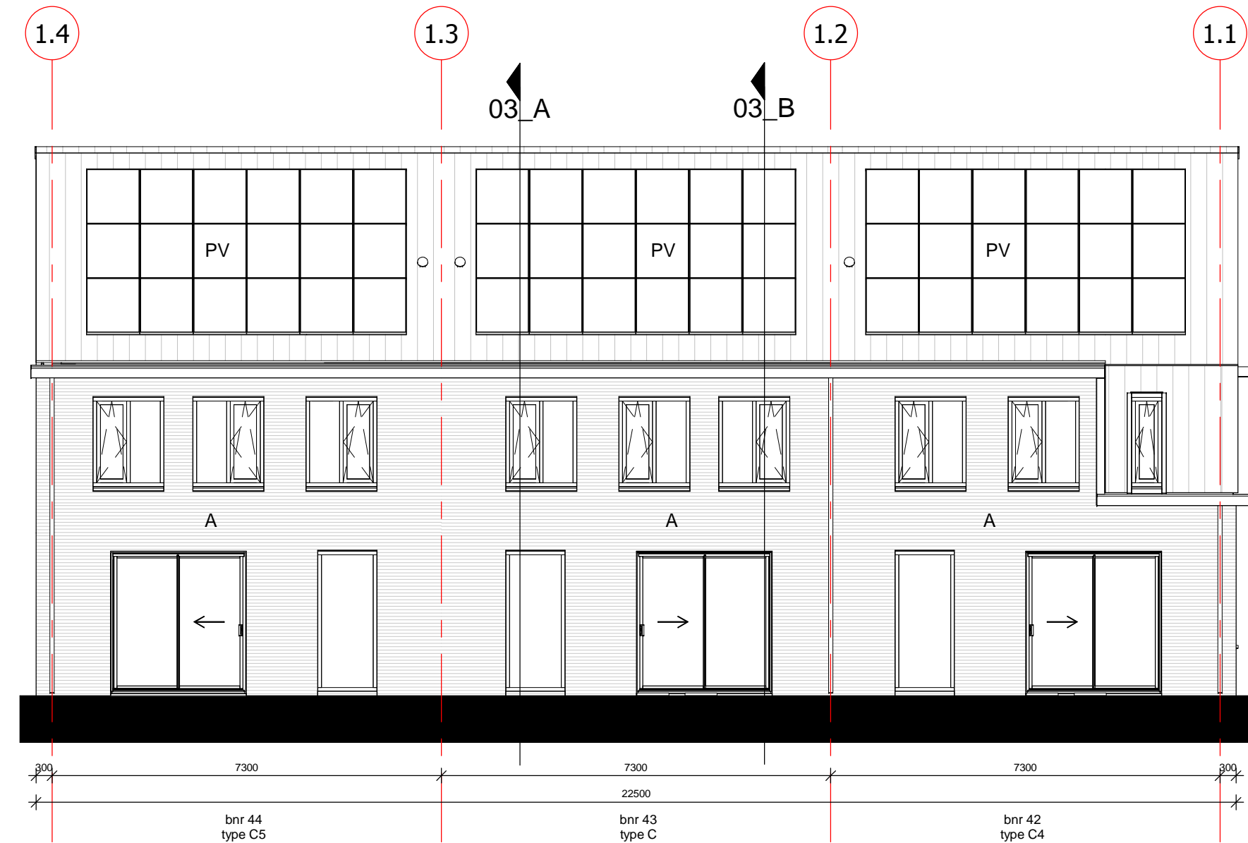
achtergevel
