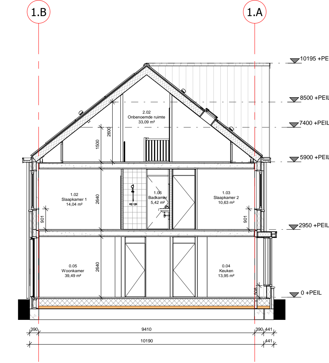
doorsnede 03_B
