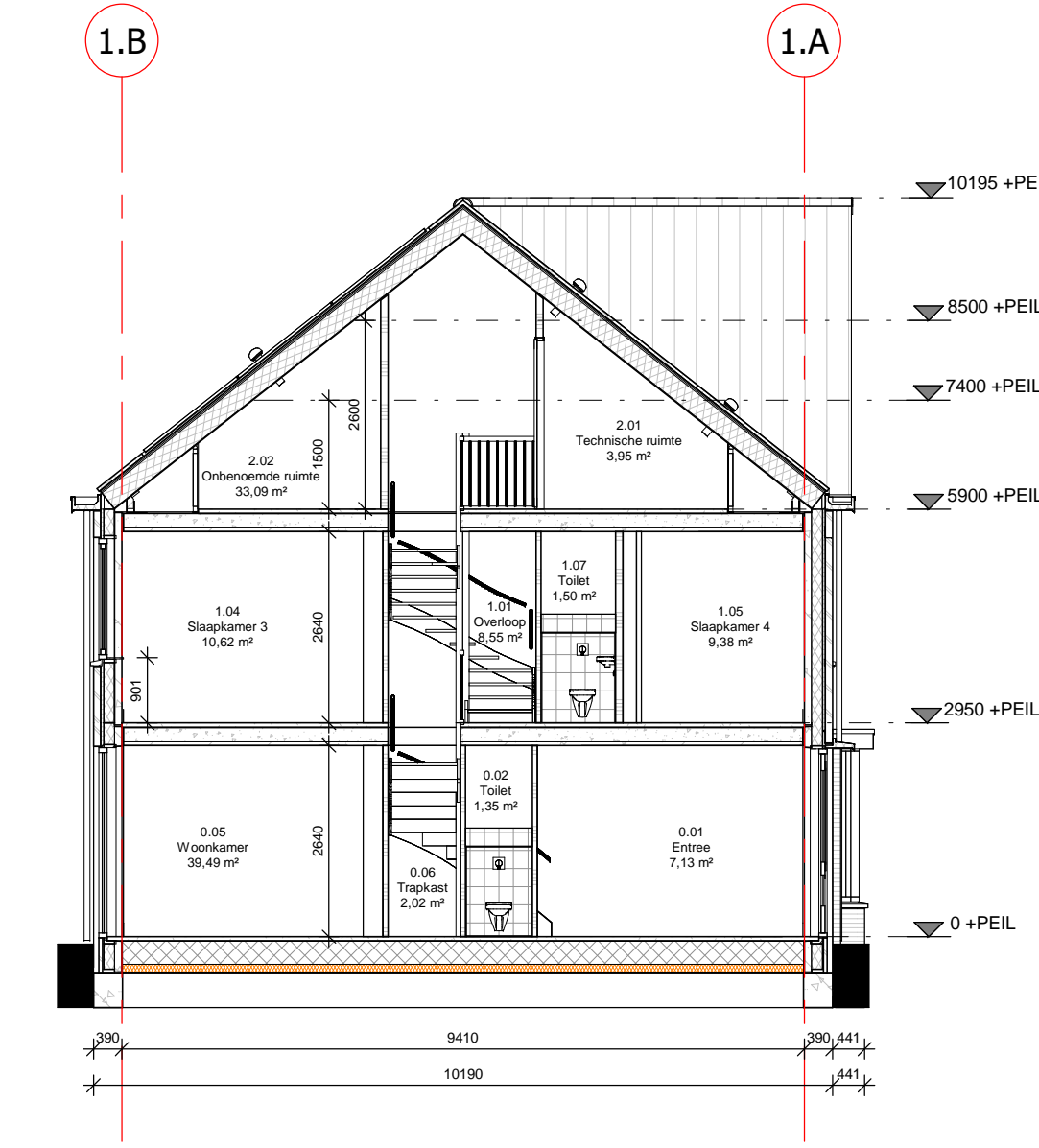
doorsnede 03_A
