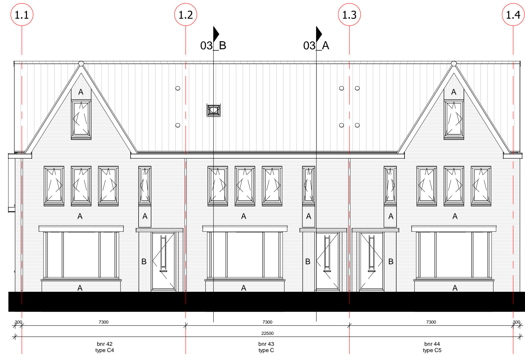
voorgevel
