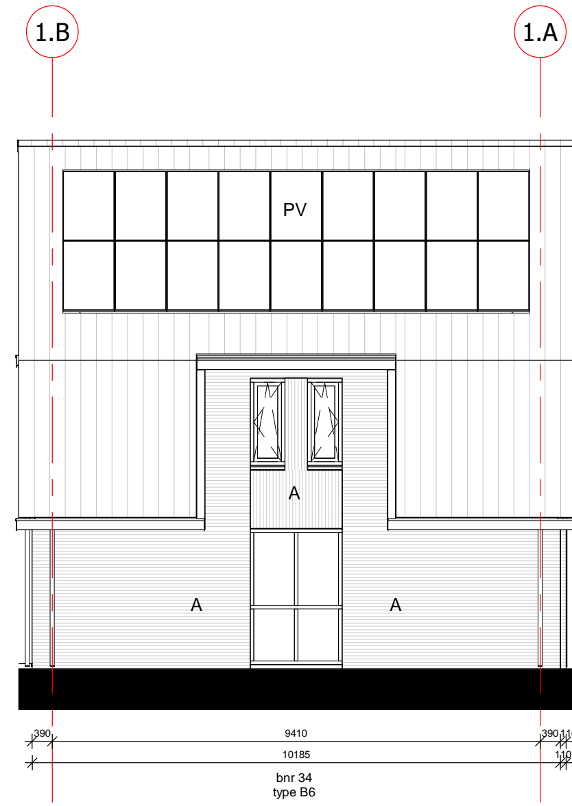
linker zijgevel
