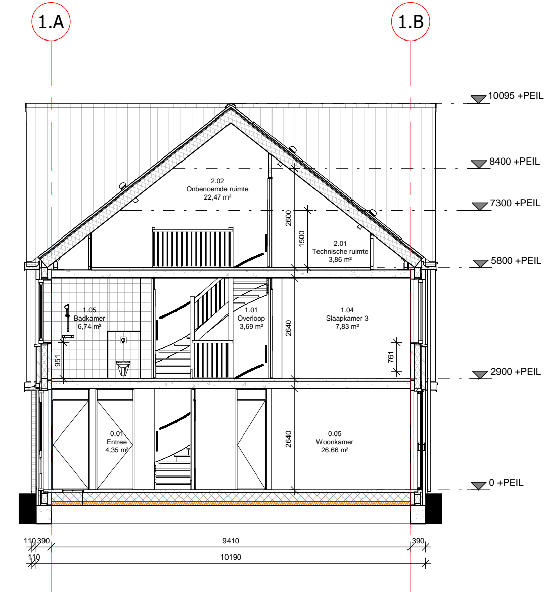
doorsnede A
