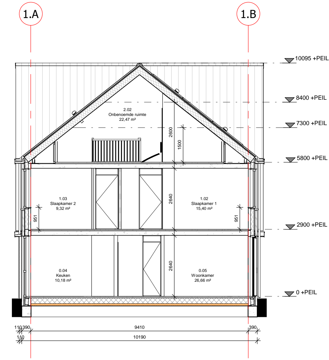
doorsnede B
