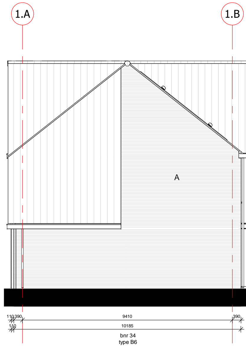
rechter zijgevel
