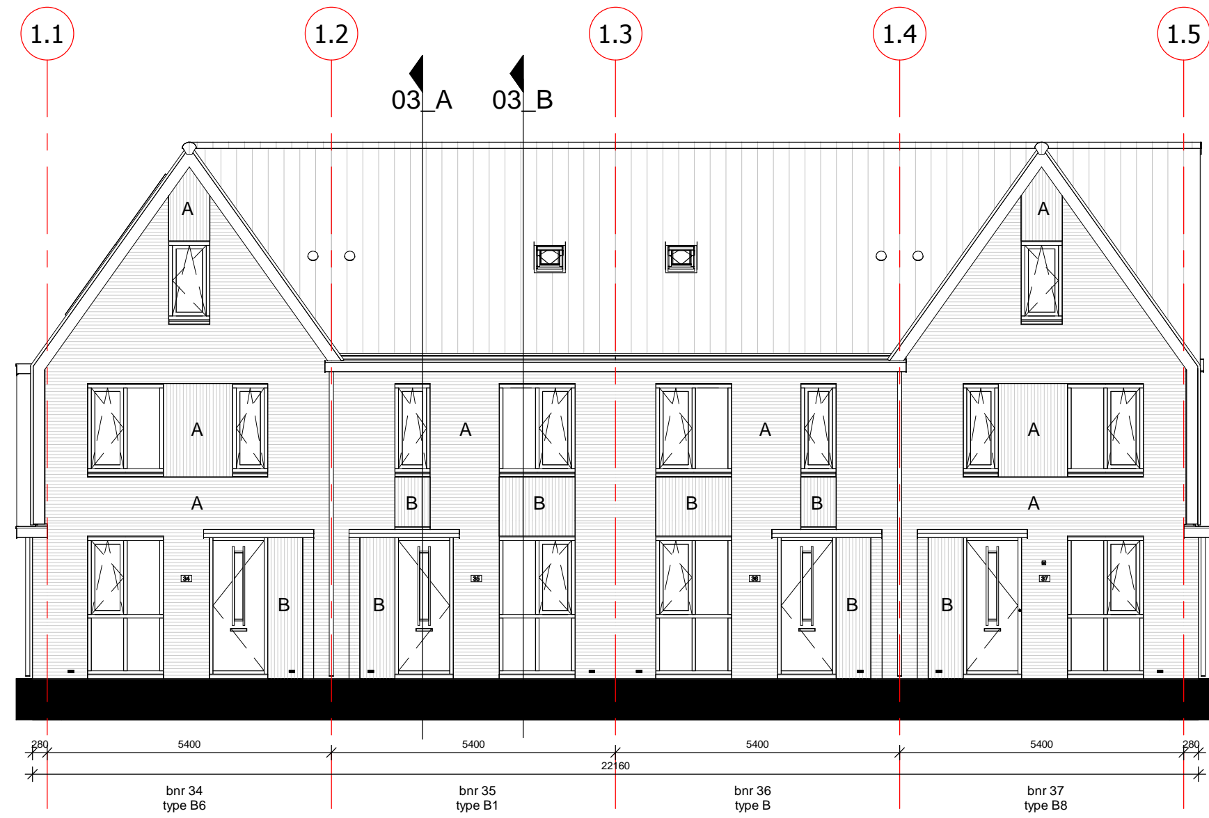
voorgevel
